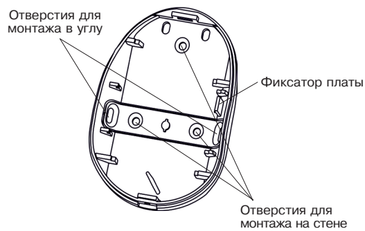
Рисунок 2 – Основание извещателя
